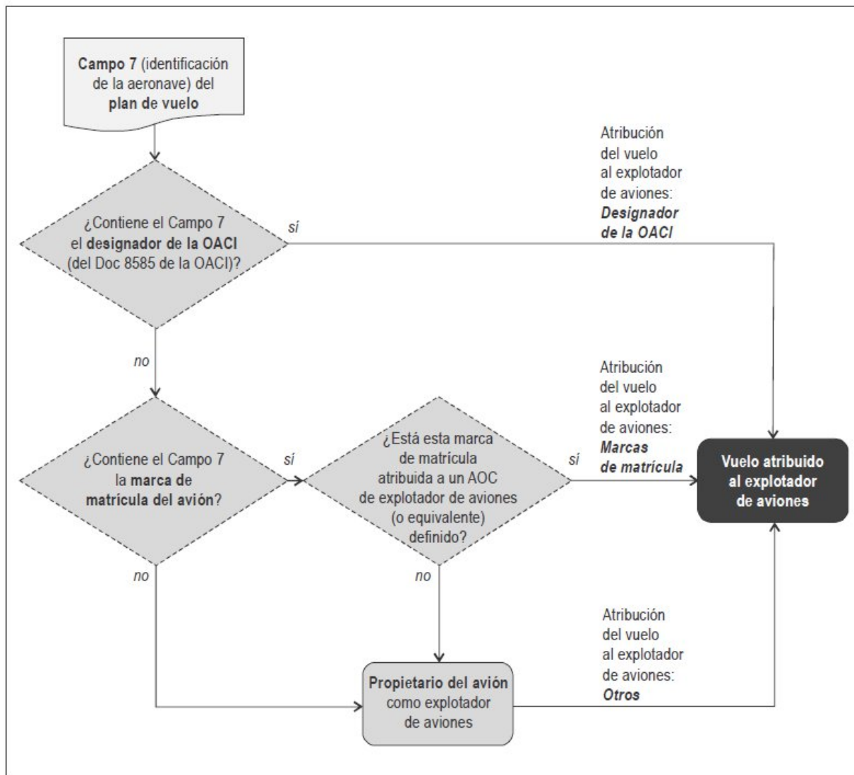
FIGURA B – 2: Proceso de atribución de un vuelo a un explotador
