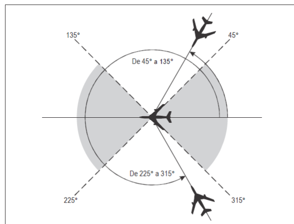
Figura 5-9 Aeronaves por derrotas que se cruzan [véase 5.4.2.1.5 c)]
