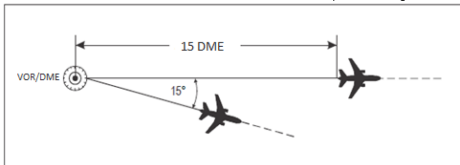
Figura 5-4.1 Separación utilizando el mismo VOR/DME [véase 5.4.1.2.1.2 a) i)]
