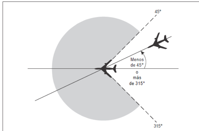
Figura 5-7 Aeronaves por la misma derrota [véase 5.4.2.1.5 a)]
