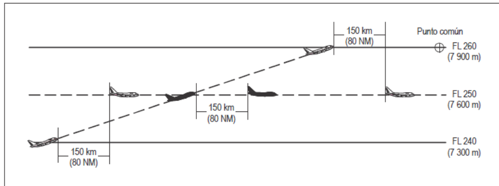
Figura 5-27A Separación de 80 NM basada en de navegación de área RNAV entre aeronaves que ascienden y por la misma derrota [véase 5.4.2.5.5 c)]
