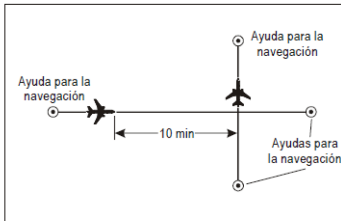
Figura 5-15 Separación de 10 minutos entre aeronaves por derrotas que se cruzan y el mismo nivel [véase 5.4.2.2.1.2 b)]
