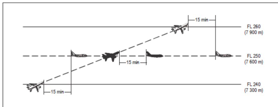
Figura 5-19A Separación de 15 minutos entre aeronaves que ascienden y por derrotras que se cruzan [véase 5.4.2.2.2.2 a)]
