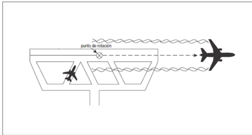
Figura 5-44 Separación por estela turbulenta para la aeronave que sigue [véanse 5.8.3.3 y 5.8.3.4]
