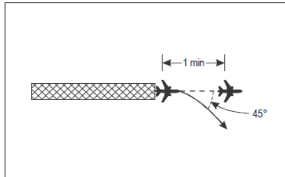
Figura 5-37 Un minuto de separación entre aeronaves que salen y siguen derrotas divergentes por lo menos en 45° [véase 5.6.1]
