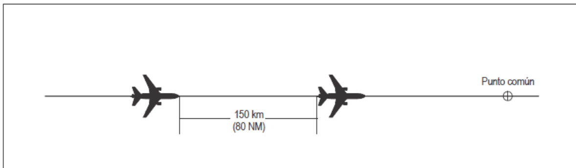
Figura 5-26 Separación de 80 NM basada en de navegación de área RNAV entre aeronaves al mismo nivel [véase 5.4.2.5.5 b)]
