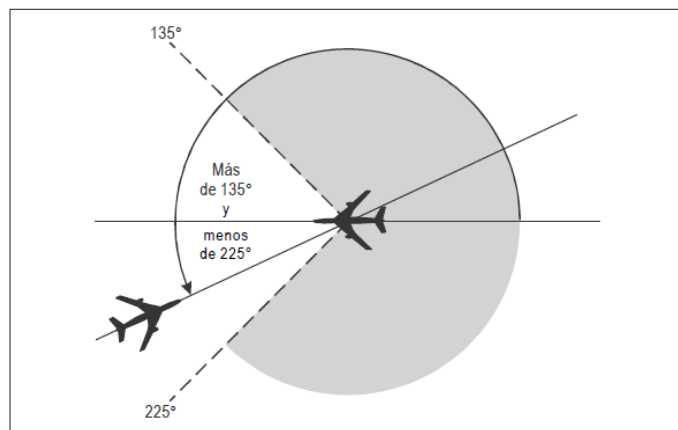
Figura 5-8 Aeronaves por derrotas opuestas [véase 5.4.2.1.5 b)]
