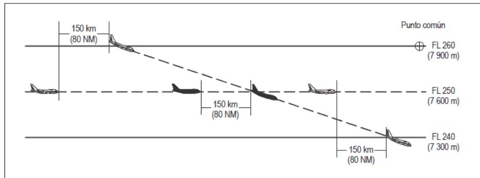
Figura 5-27B Separación de 80 NM basada en de navegación de área RNAV entre aeronaves que descienden y por la misma derrota [véase 5.4.2.5.5 c)]
