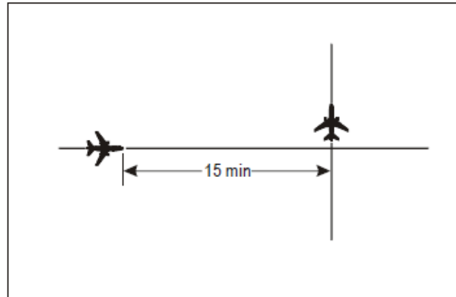
Figura 5-14 Separación de 15 minutos entre aeronaves por derrotas que se cruzan y el mismo nivel [véase 5.4.2.2.1.2 a)]
