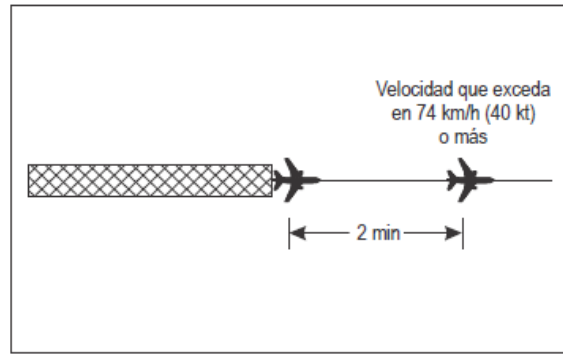
Figura 5-38 Dos minutos de separación entre aeronaves que salen y siguen la misma derrota [véase 5.6.2]
