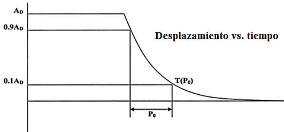
Figura 3.2B Respuesta al movimiento momentáneo de un sistema crítico o de alta amortiguación.
