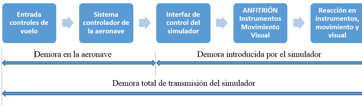
Figura 3.2F Tiempos de transmisión para simulación de aeronaves controladas por computador usando cajas negras reales de helicóptero
