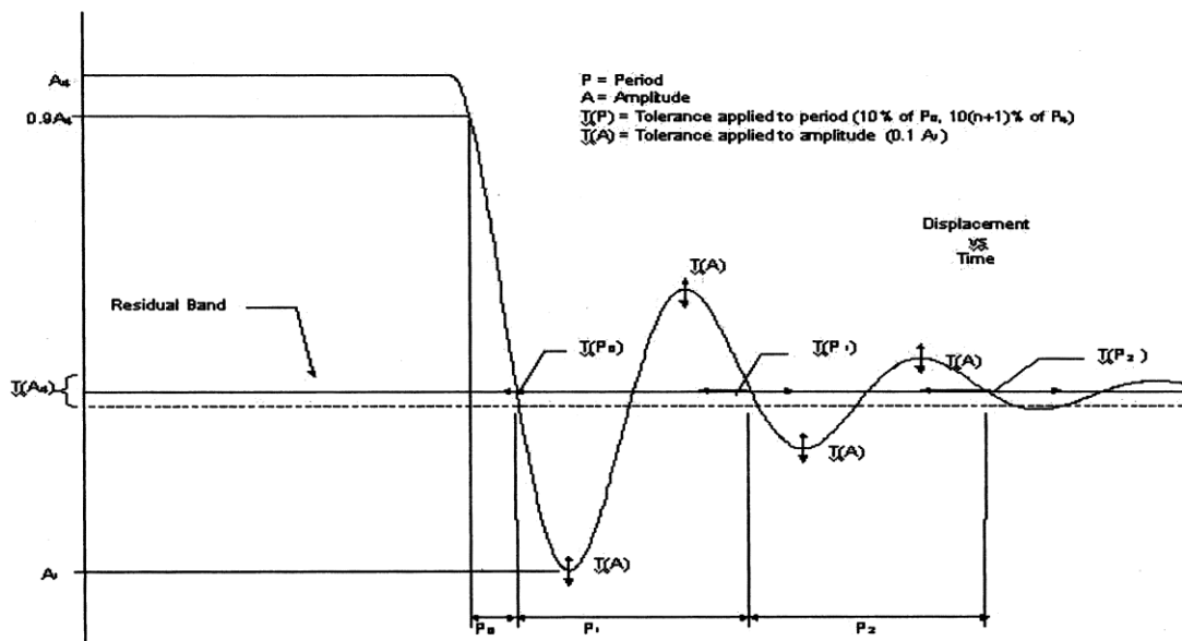
Figura 1-IIA - Respuesta al movimiento momentáneo de un sistema de baja amortiguación
