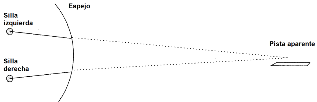
Figura 3.2J Visualización de la pista en una pantalla colimada
