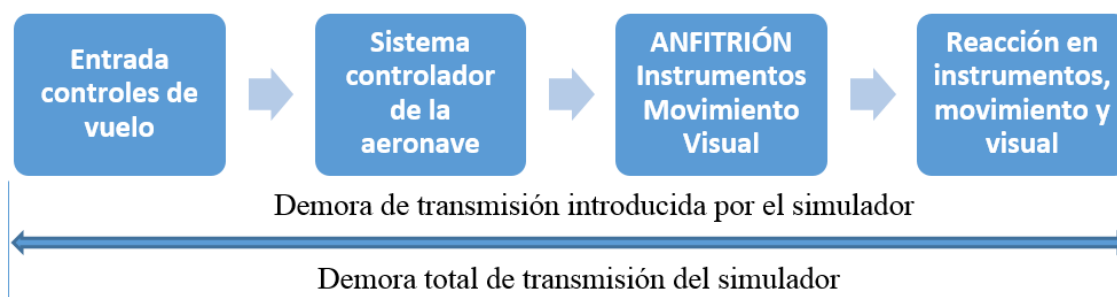
Figura 3.2E Tiempos de transmisión para simulación de aeronaves clásicas no controladas por computador
