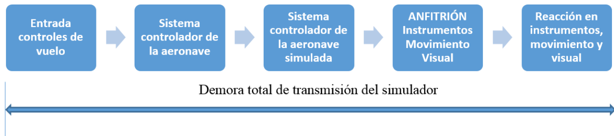
Figuras 3.2HA y 3.2HB Tiempos de transmisión para simulación de helicópteros usando controladores de instrumento reales o reconfigurados
