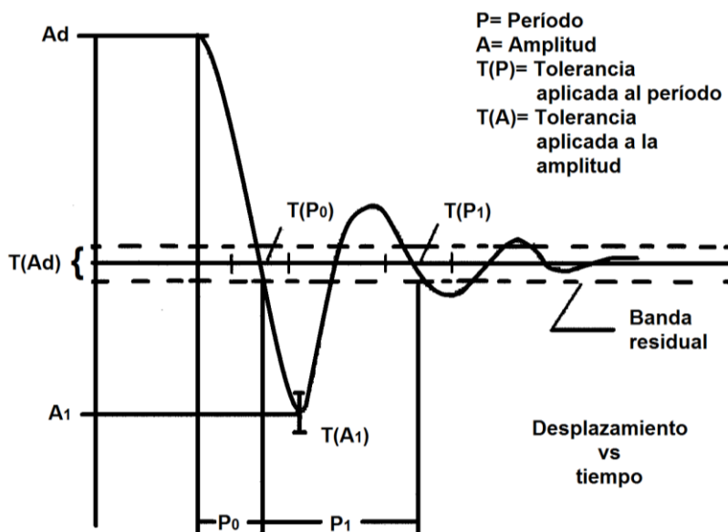
Figura 4.2A Respuesta con amortiguación
