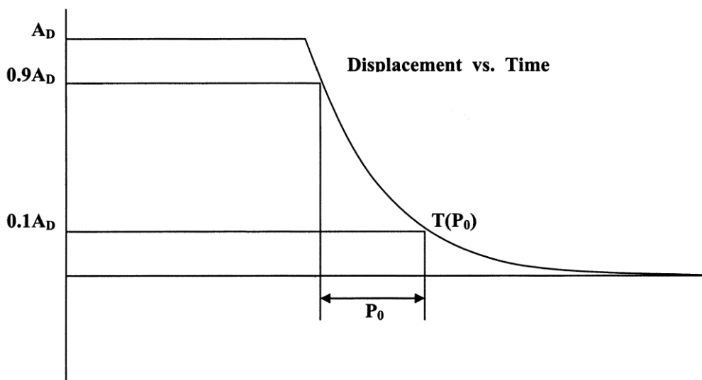
Figura 1-II2B - Respuesta al movimiento momentáneo de un sistema crítico o de alta amortiguación
