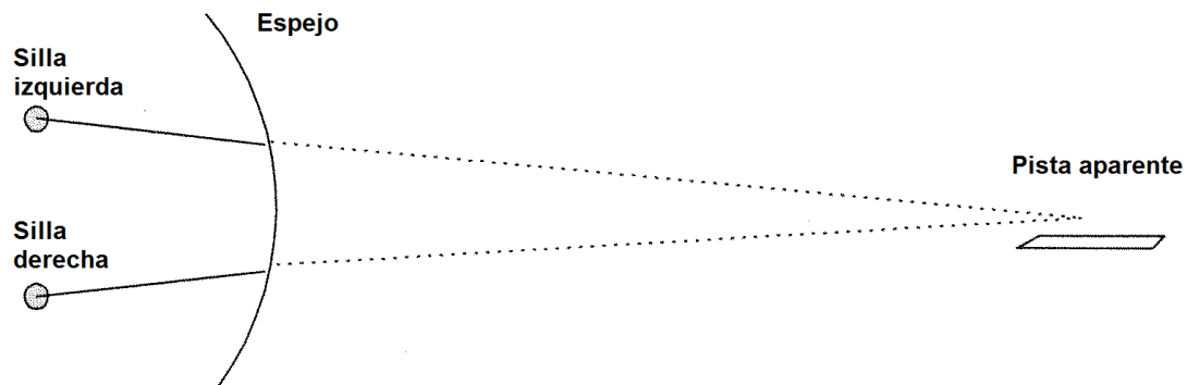
Figura 3.2J Visualización de la pista en una pantalla colimada
