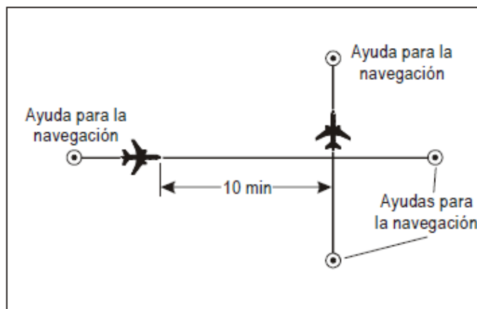
Figura 5-15 Separación de 10 minutos entre aeronaves por derrotras que se cruzan y el mismo nivel
