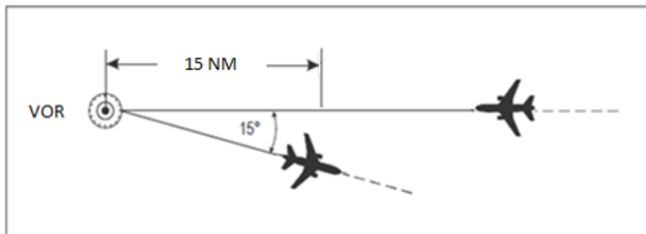
Figura 5-4.6 Separación utilizando el mismo VOR [véase 5.4.1.2.1.2 a) vi)]
