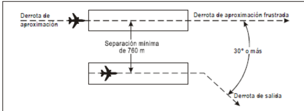
Figura 6-7. Operaciones paralelas segregadas [véase 6.7.3.6.1 b)]
