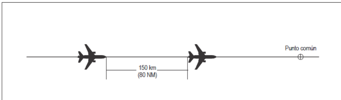
Figura 5-26 Separación de 80 NM basada en RNAV entre aeronaves al mismo nivel [véase 5.4.2.5.5 b)]
