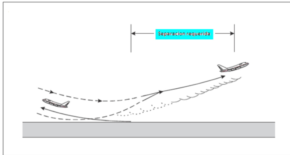
Figura 5-45 Separación por estela turbulenta para despegue en sentidos opuestos [véanse 5.8.5.1 a) y 5.8.5.2 a)]
