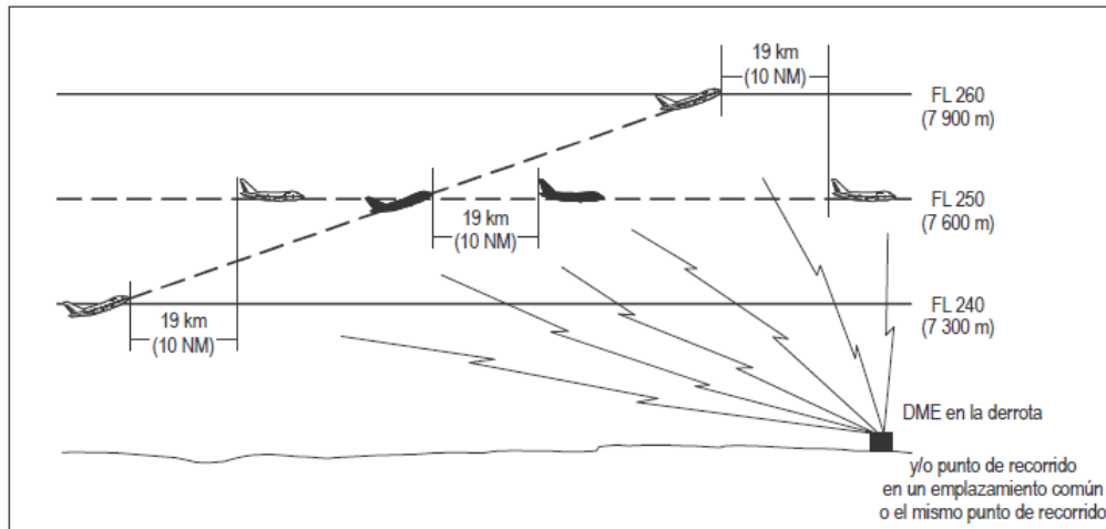
Figura 5-25A. Separación de 10 NM basada en DME o GNSS entre aeronaves que ascienden y por la misma derrota [véase 5.4.2.3.4.1 c)]
