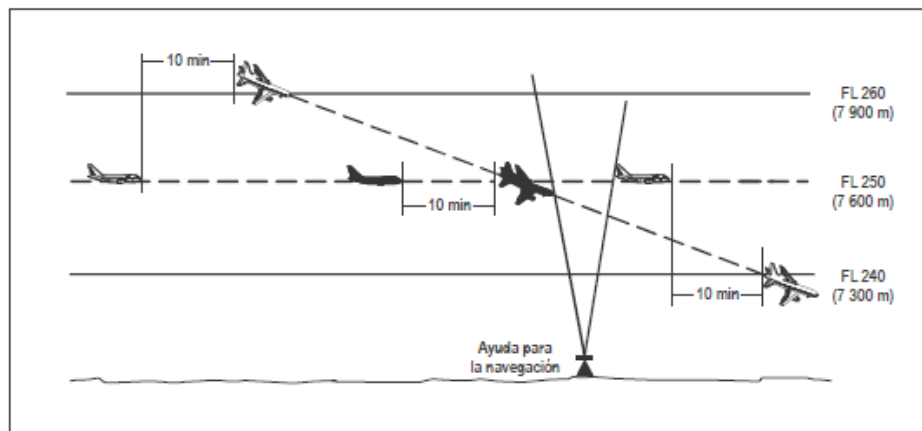
Figura 5-20B Separación de 10 minutos entre aeronaves que descienden y por derrotas que se cruzan [véase 5.4.2.2.2.2 b)]
