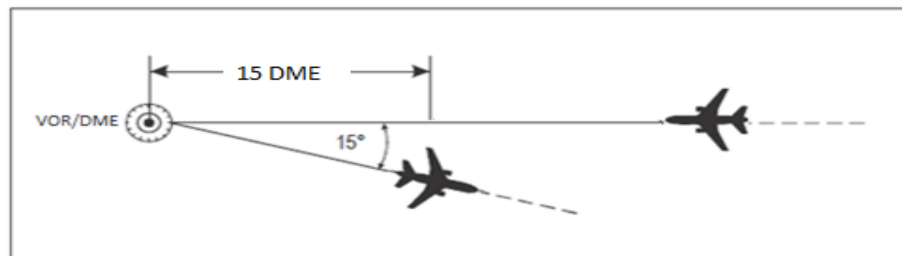
Figura 5-4.3 Separación utilizando el mismo VOR/DME [véase 5.4.1.2.1.2 a) iii)]
