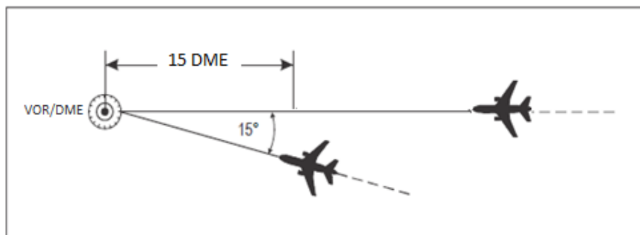
Figura 5-4.2 Separación utilizando el mismo VOR/DME [véase 5.4.1.2.1.2 a) ii)]
