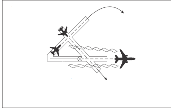
Figura 5-43 Separación por estela turbulenta para aeronaves que se cruzan [véanse 5.8.3.1 b) y 5.8.3.2 b)]
