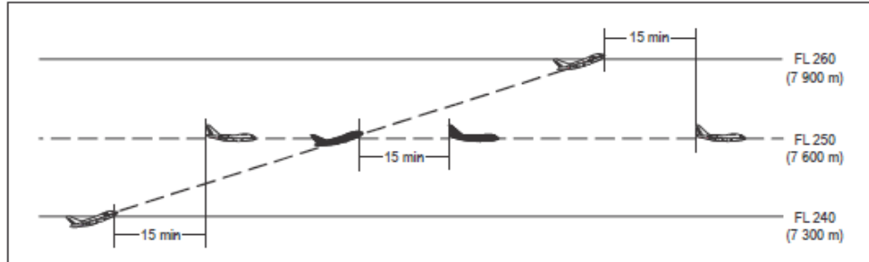
Figura 5-16A Separación de 15 minutos entre aeronaves que ascienden y por la misma derrota [véase 5.4.2.2.2.1 a)]
