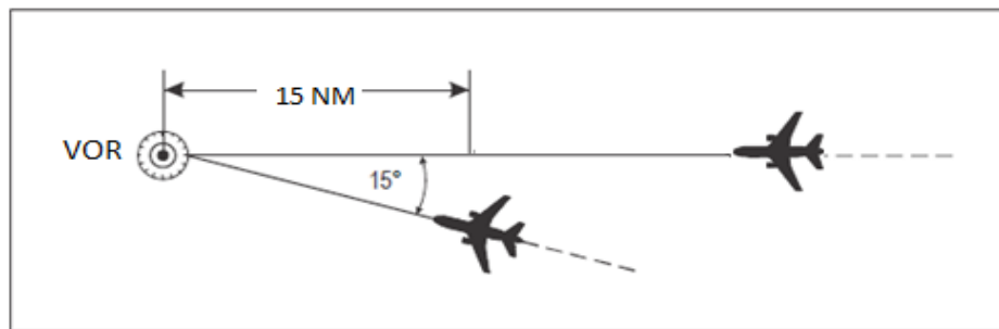
Figura 5-4.5 Separación utilizando el mismo VOR [véase 5.4.1.2.1.2 a) v)]
