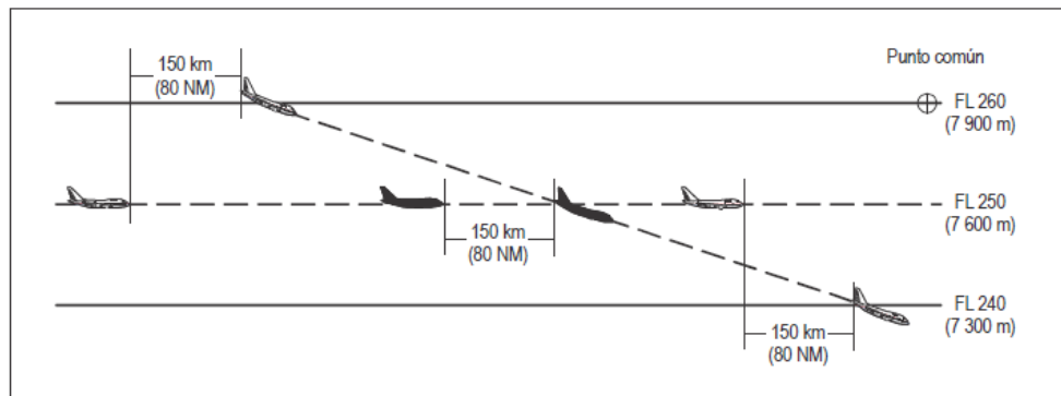
Figura 5-27B Separación de 80 NM basada en RNAV entre aeronaves que descienden y por la misma derrota [véase 5.4.2.5.5 c)]
