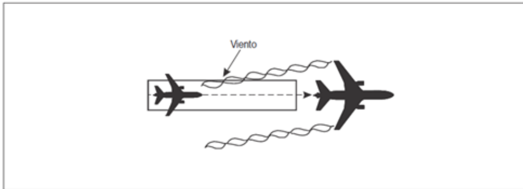
Figura 5-42 Separación por estela turbulenta para aeronaves que siguen [véanse 5.8.3.1 a), y 5.8.3.2 a)]
