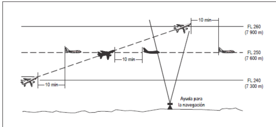
Figura 5-20A Separación de 10 minutos entre aeronaves que ascienden y por derrotas que se cruzan [véase 5.4.2.2.2.2 b)]
