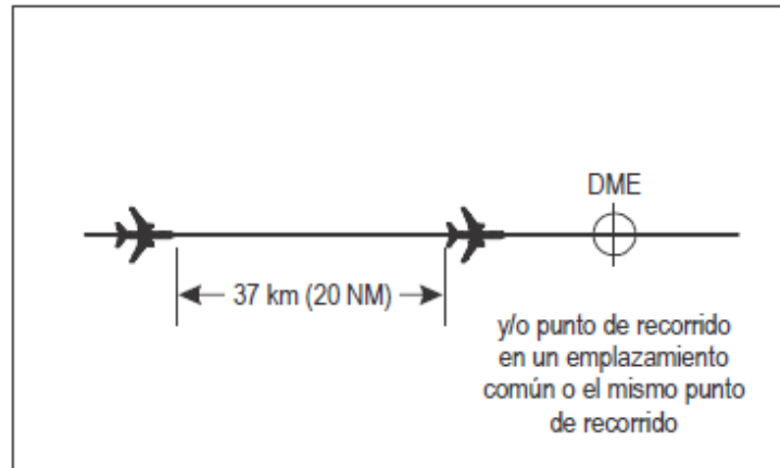
Figura 5-22. Separación de 20NM basada en DME o GNSS entre aeronaves por la misma derrota y al mismo nivel [véase 5.4.2.3.3.1 a)]
