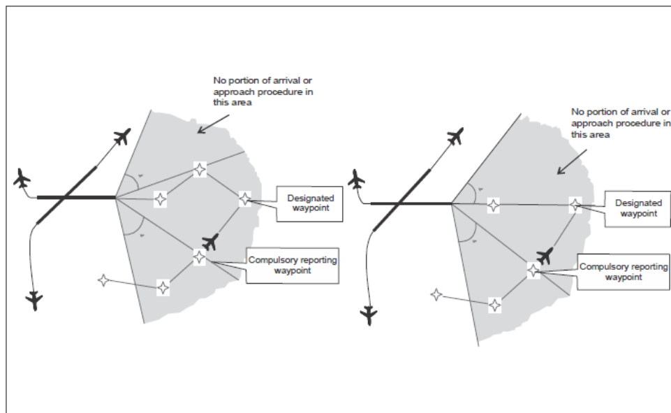
Figura 5-41. Área de protección de llegada
