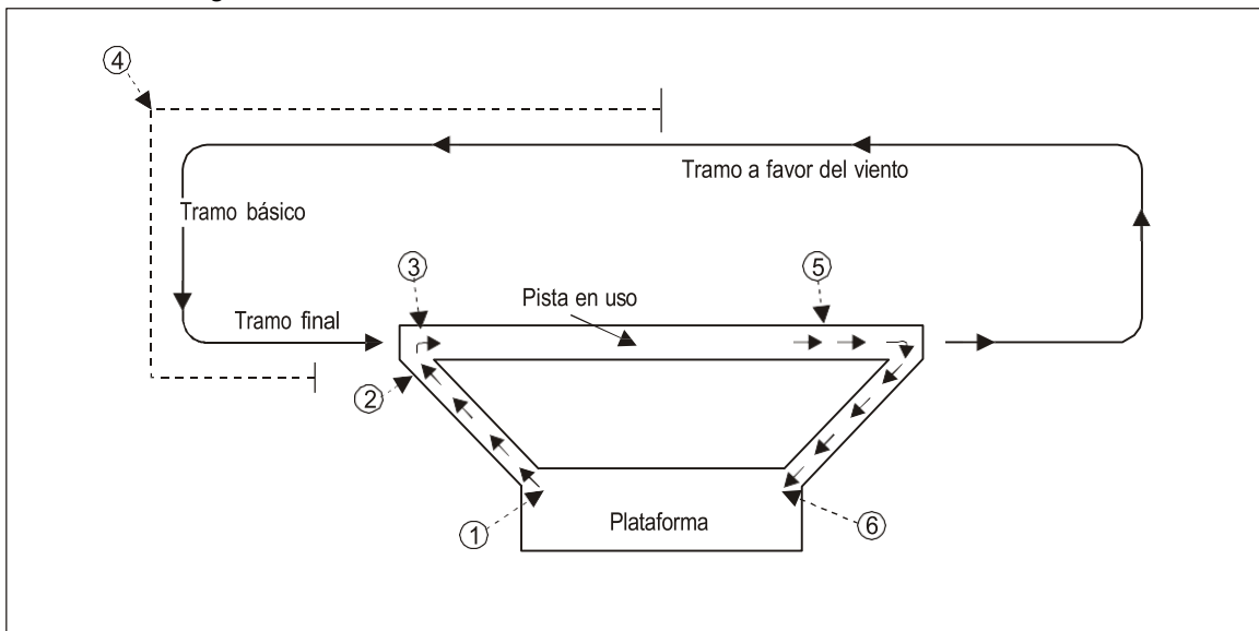
Figura 7-1. Posiciones designadas de las aeronaves desde un punto de vista de la torre de control de aeródromo (véase 7.6.2)
