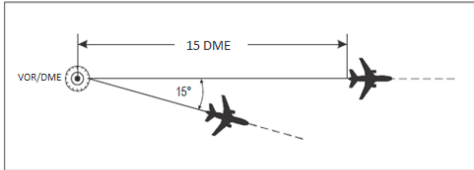
Figura 5-4.1 Separación utilizando el mismo VOR/DME [véase 5.4.1.2.1.2 a) i)]
