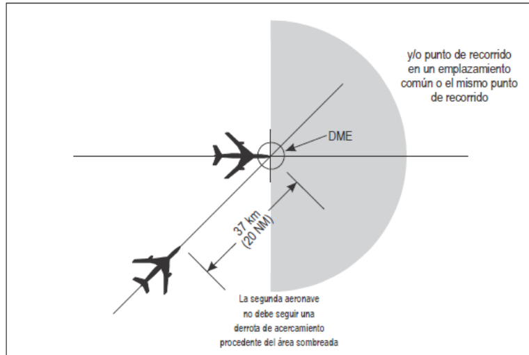
Figura 5-24A. Separación de 20NM basada en DME o GNSS entre aeronaves por derrotas que se cruzan y al mismo nivel (véase 5.4.2.3.3.2)
