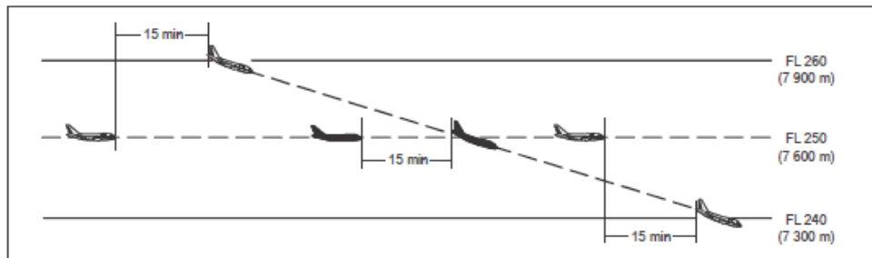
Figura 5-16B Separación de 15 minutos entre aeronaves que descienden y por la misma derrota [véase 5.4.2.2.2.1 a)]
