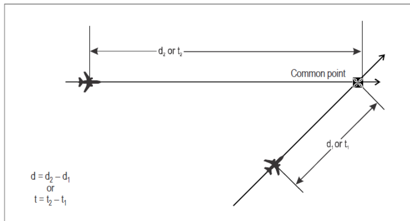
Figura 5-33. Cálculo de la distancia/tiempo longitudinal entre aeronaves - misma derrota prevista, pero no idéntica [véase 5.4.2.9.5 b)]
