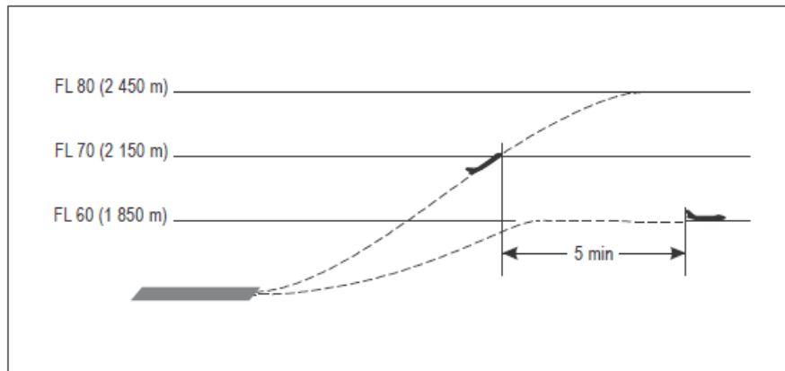
Figura 5-39 Cinco (5) minutos de separación entre aeronaves que salen siguiendo la misma derrota [véase 5.6.3]
