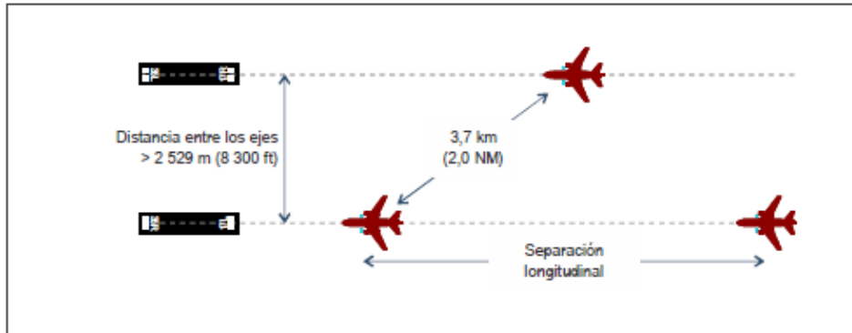
Figura 6-3. Separación diagonal para una distancia entre ejes mayor que 2 529 m (8 300 ft)
