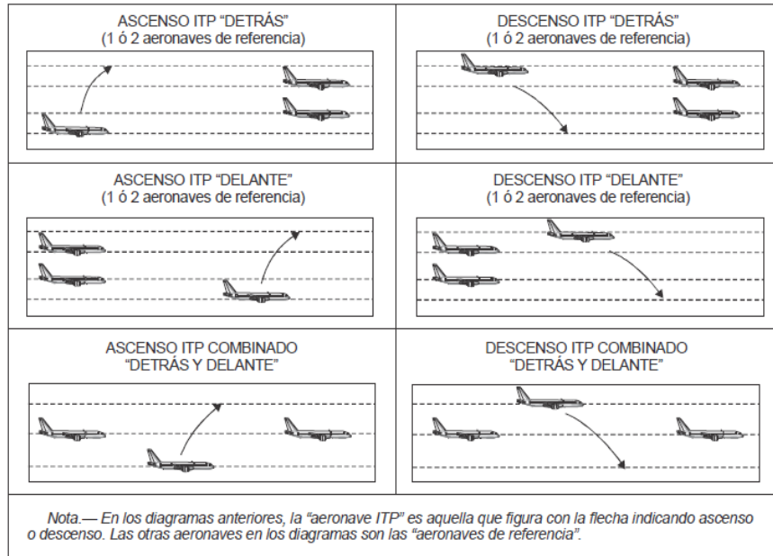
Figura 5-29 Escenarios de cambio de nivel de vuelo IT [véase 5.4.2.7.3]
