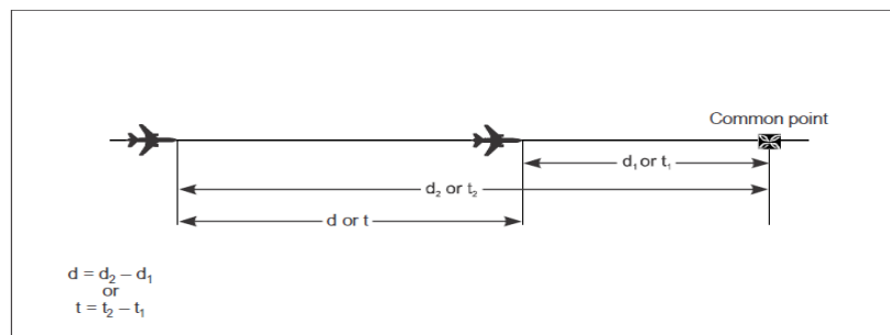
Figura 5-30. Cálculo de la distancia/tiempo longitudinal entre aeronaves - derrota idéntica, mismo sentido [véase 5.4.2.9.5 a)]
