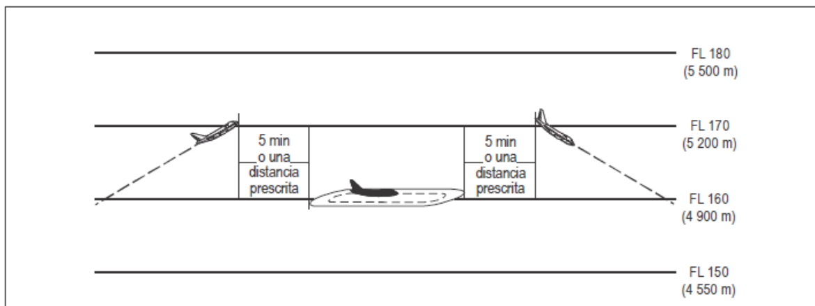
Figura 5-36 Separación entre aeronaves en circuito de espera y aeronaves en ruta [5.5.2]
