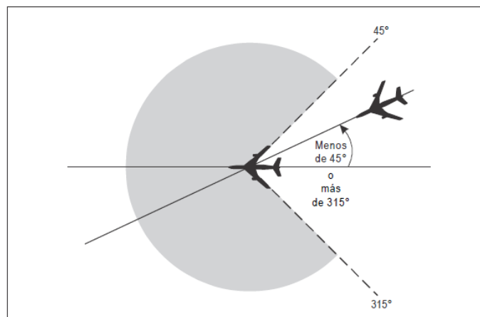
Figura 5-7 Aeronaves por la misma derrota [véase 5.4.2.1.5 a)]
