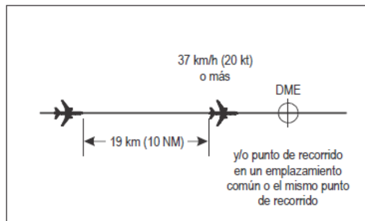
Figura 5-23. Separación de 10NM basada en DME o GNSS entre aeronaves por la misma derrota y al mismo nivel [véase 5.4.2.3.3.1 b)]
