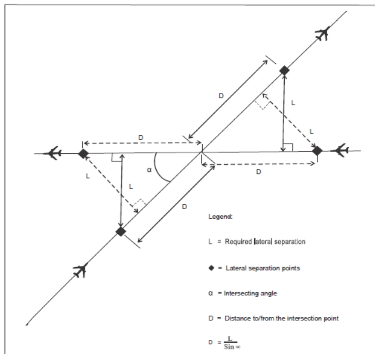
Figura 5-6 Puntos de separación lateral (véase 5.4.1.2.1.7)
