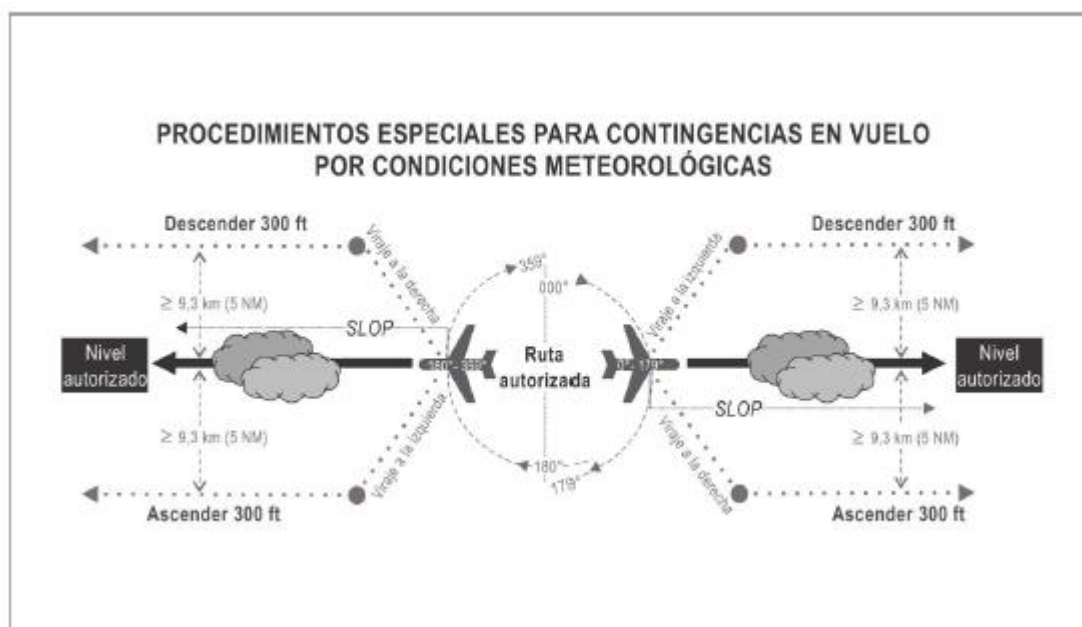
Figura 15-2. Guía visual de los procedimientos para desviarse por condiciones meteorológicas si no se puede obtener una autorización revisada del ATC (véase 15.2.4.3)
