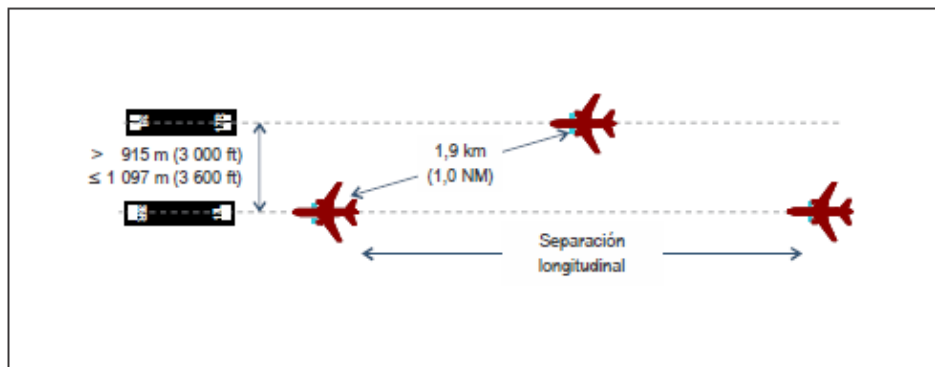
Figura 6-5. Separación diagonal para una distancia entre ejes mayor que 915 m (3 000 ft) pero menor o igual a 1 097 m (3 600 ft)
