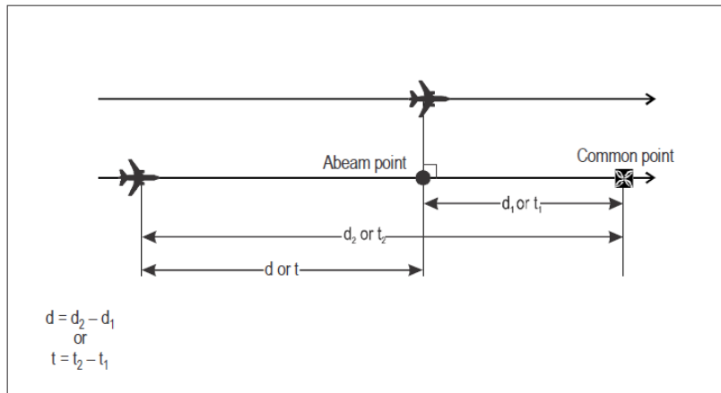
Figura 5-35. Cálculo de la distancia/tiempo longitudinal entre aeronaves - derrota paralelas [véase 5.4.2.9.5 c)]
