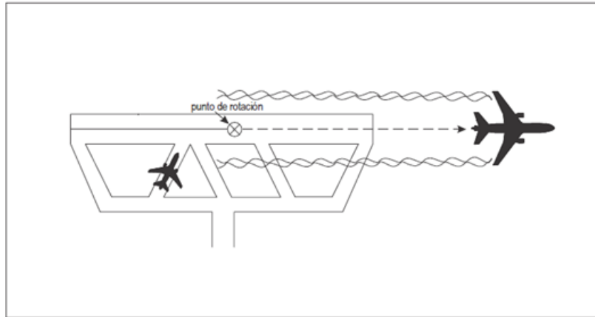
Figura 5-44 Separación por estela turbulenta para la aeronave que sigue [véanse 5.8.3.3 y 5.8.3.4]
