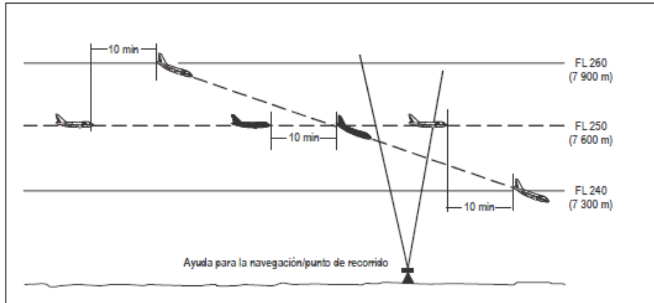
Figura 5-17B Separación de 10 minutos entre aeronaves que descienden y por la misma derrota [véase 5.4.2.2.2.1 b)]
