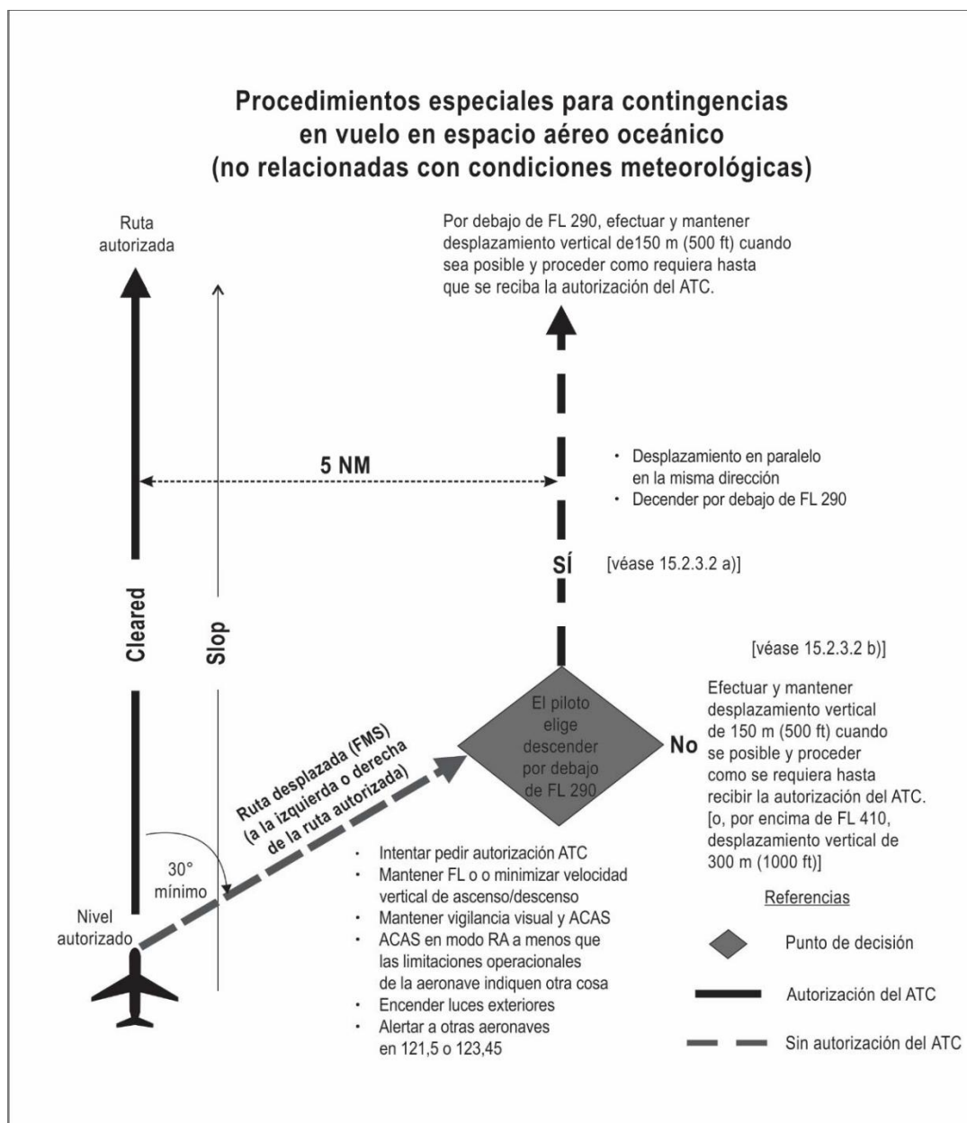
Figura 15-1. Guía visual de procedimientos en caso de contingencia (véanse los puntos 15.2.2 y 15.2.3)
