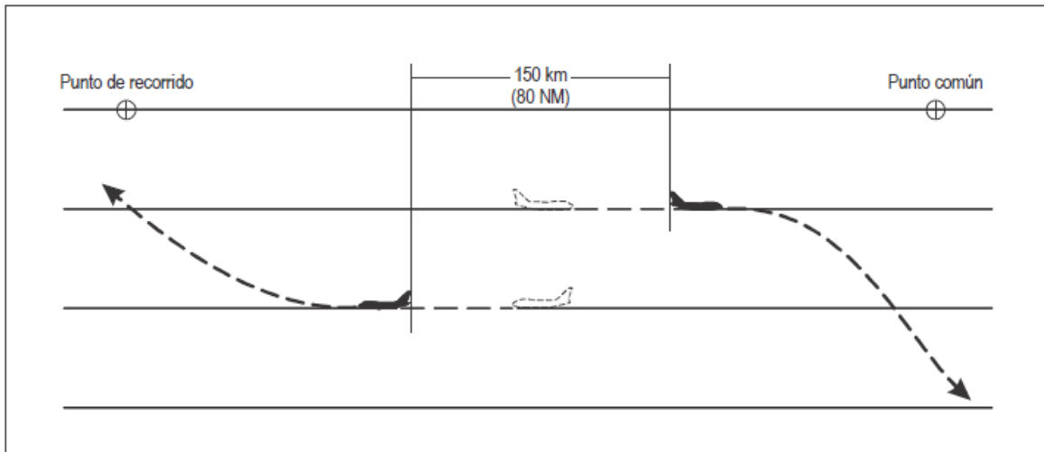
Figura 5-28 Separación de 80 NM basada en RNAV entre aeronaves por derrotas opuestas [véase 5.4.2.5.7]
