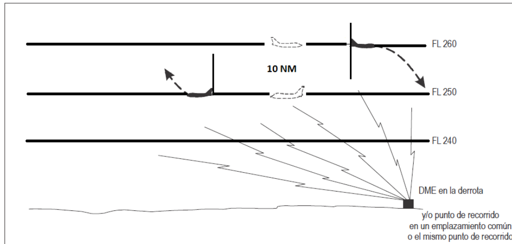
Figura 5-25C. Separación de 10 NM basada en DME o GNSS entre aeronaves que siguen derrotas opuestas [véase 5.4.2.3.4.2)
