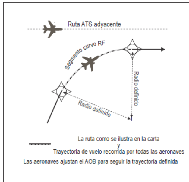
Figura 5-2. Viraje de transición de radio fijo (FRT) y con arco de radio constante hasta un punto de referencia (RF) (véase 5.4.1.1.4)
