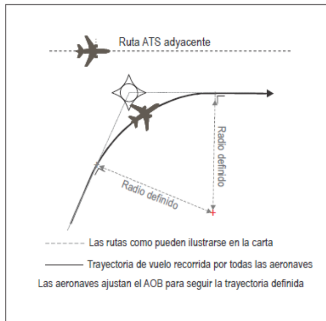
Figura 5-1 (cont.). Viraje sobre un punto de recorrido de sobrevuelo y viraje en un punto de recorrido de paso (véase 5.4.1.1.4)
