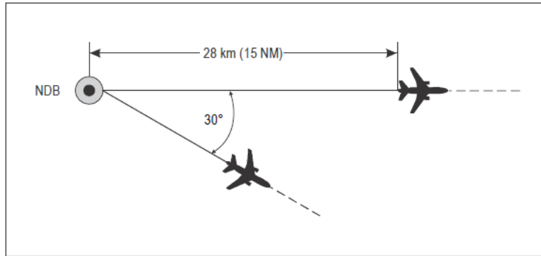
Figura 5-5 Separación utilizando el mismo NDB [véase 5.4.1.2.1.2 b)]
