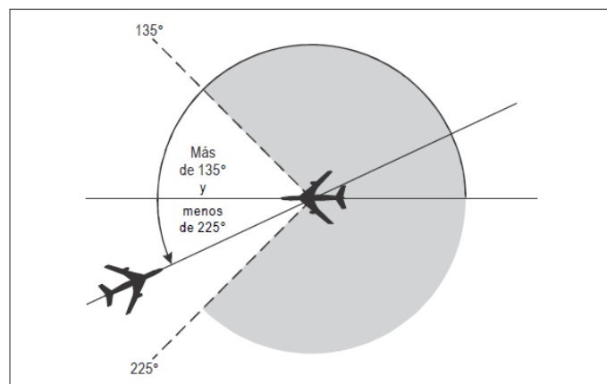
Figura 5-8 Aeronaves por derrota opuesta [véase 5.4.2.1.5 b)]
