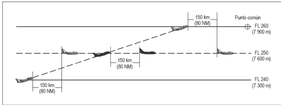
Figura 5-27A Separación de 80 NM basada en RNAV entre aeronaves que ascienden y por la misma derrota [véase 5.4.2.5.5 c)]
