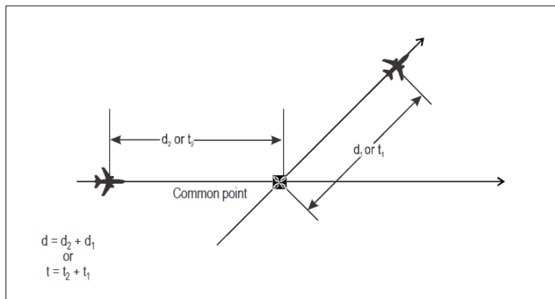
Figura 5-34. Cálculo de la distancia/tiempo longitudinal entre aeronaves - lados opuestos del punto común [véase 5.4.2.9.5 b)]
