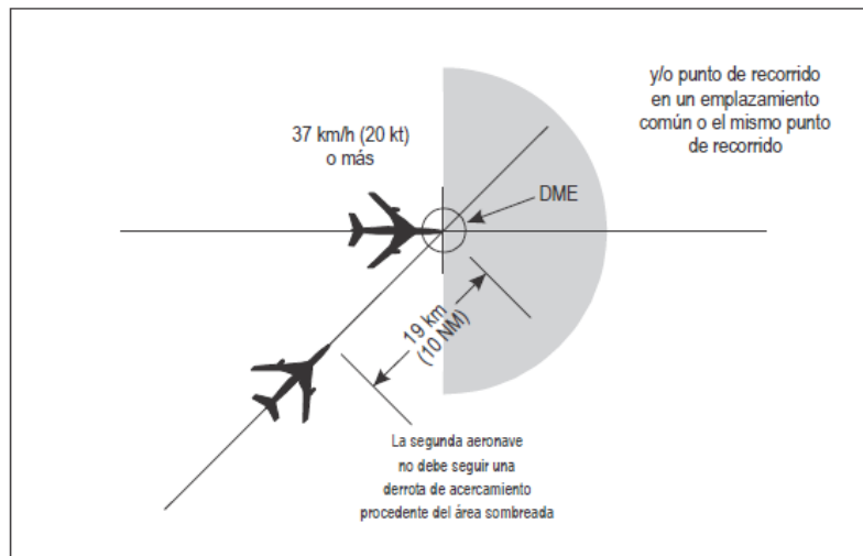
Figura 5-24B. Separación de 10NM basada en DME o GNSS entre aeronaves por derrotas que se cruzan y al mismo nivel (véase 5.4.2.3.3.2)
