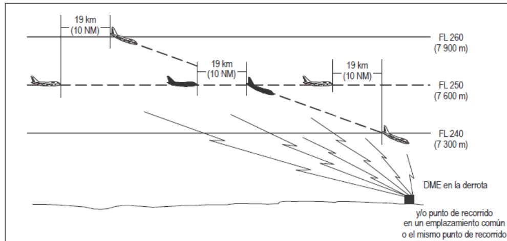
Figura 5-25B. Separación de 10 NM basada en DME o GNSS entre aeronaves que descienden y por la misma derrota [véase 5.4.2.3.4.1 c)]
