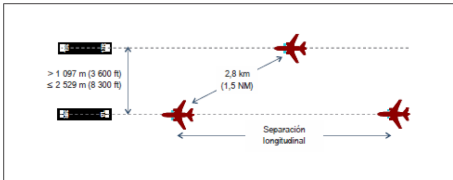
Figura 6-4. Separación diagonal para una distancia entre ejes mayor que 1 097 m (3 600 ft), pero menor o igual a 2 529 m (8 300 ft)
