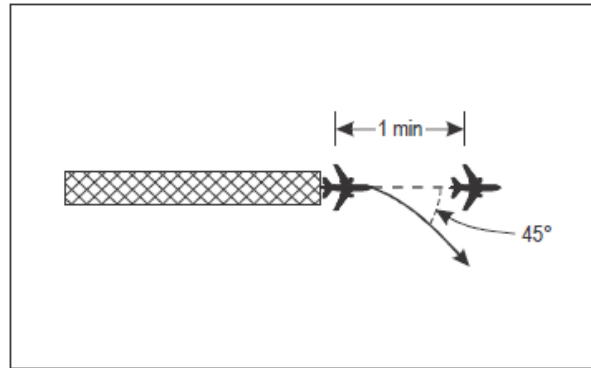
Figura 5-37 Un minuto de separación entre aeronaves que salen y siguen derrota divergentes por lo menos en 45° [véase 5.6.1]
