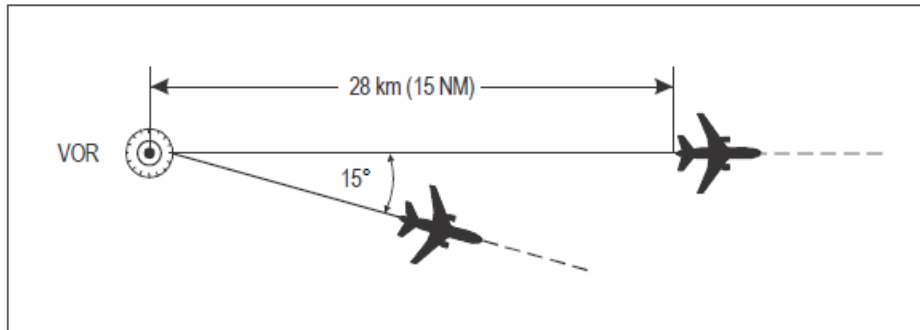
Figura 5-4.4 Separación utilizando el mismo VOR [véase 5.4.1.2.1.2 a) iv)]
