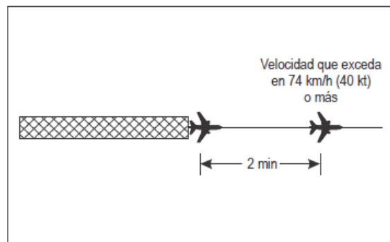
Figura 5-38 Dos minutos de separación entre aeronaves que salen y siguen la misma derrota [véase 5.6.2]
