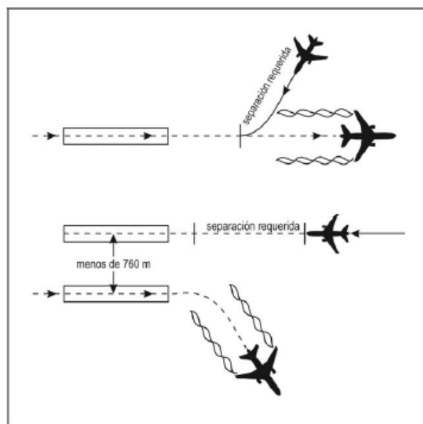
Figura 5-46 Separación por estela turbulenta para aterrizaje en sentidos opuestos [véanse 5.8.5.1 b) y 5.8.5.2 b)]
