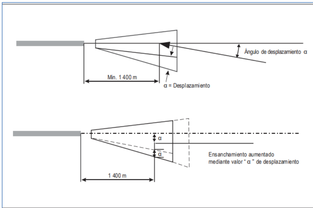
Figura 10-1. Vista en planta de superficie de tramo visual para aproximación final desplazada que cruza el eje de la pista
