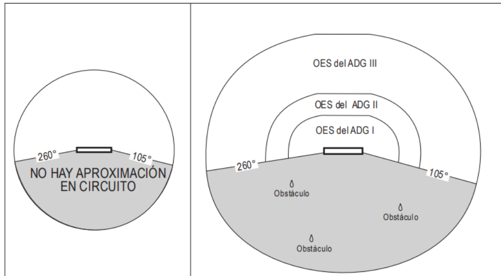
Figura 10-2. Modificación de la OES horizontal en un área que no sea de aproximación en circuito
