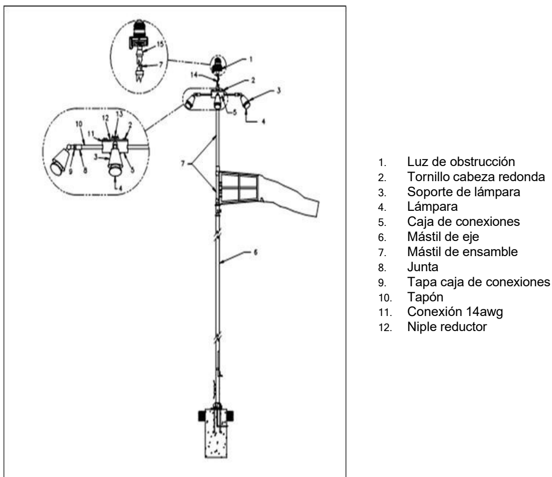
Figura 2-7-1. Indicador de dirección del viento iluminado
