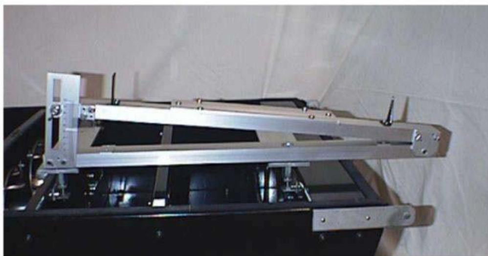
Figura 2-8-1. Detalle del elemento de ajuste del ángulo de la unidad PAPI
