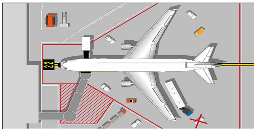
Figura 10. Ningún vehículo debe estacionarse al frente de vehículo de reabastecimiento de combustible impidiendo su circulación inmediata.
