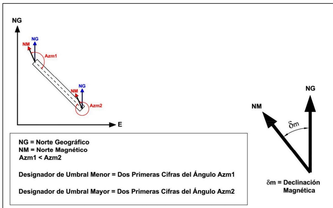
Figura A8-4.- Esquema explicativo para determinación de designador de umbral.
