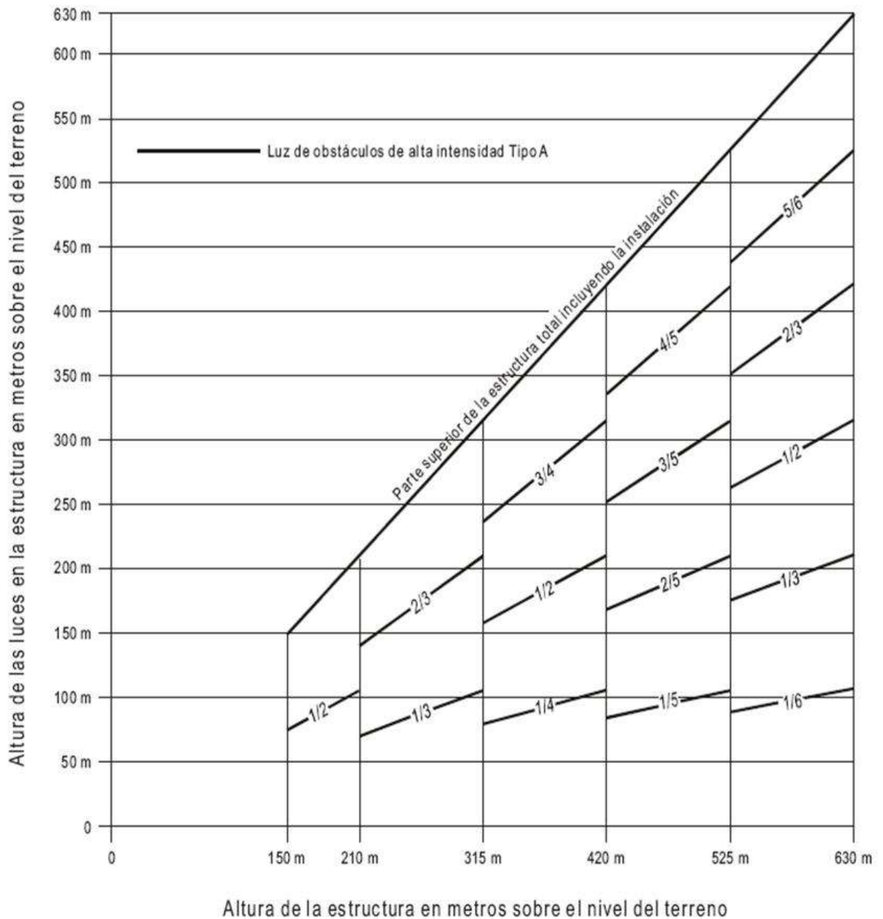
Figura A6-6. Sistema de iluminación de obstáculos con luces blancas de destellos de alta intensidad de Tipo A
