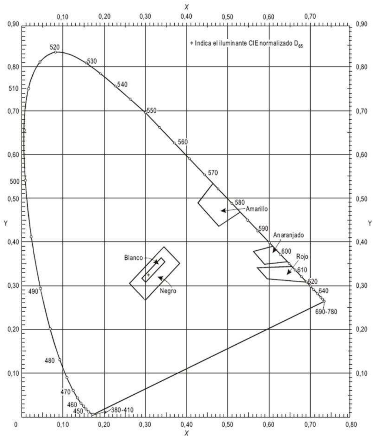
Figura A1-2. Colores ordinarios para las señales y los letreros y tableros con iluminación externa
