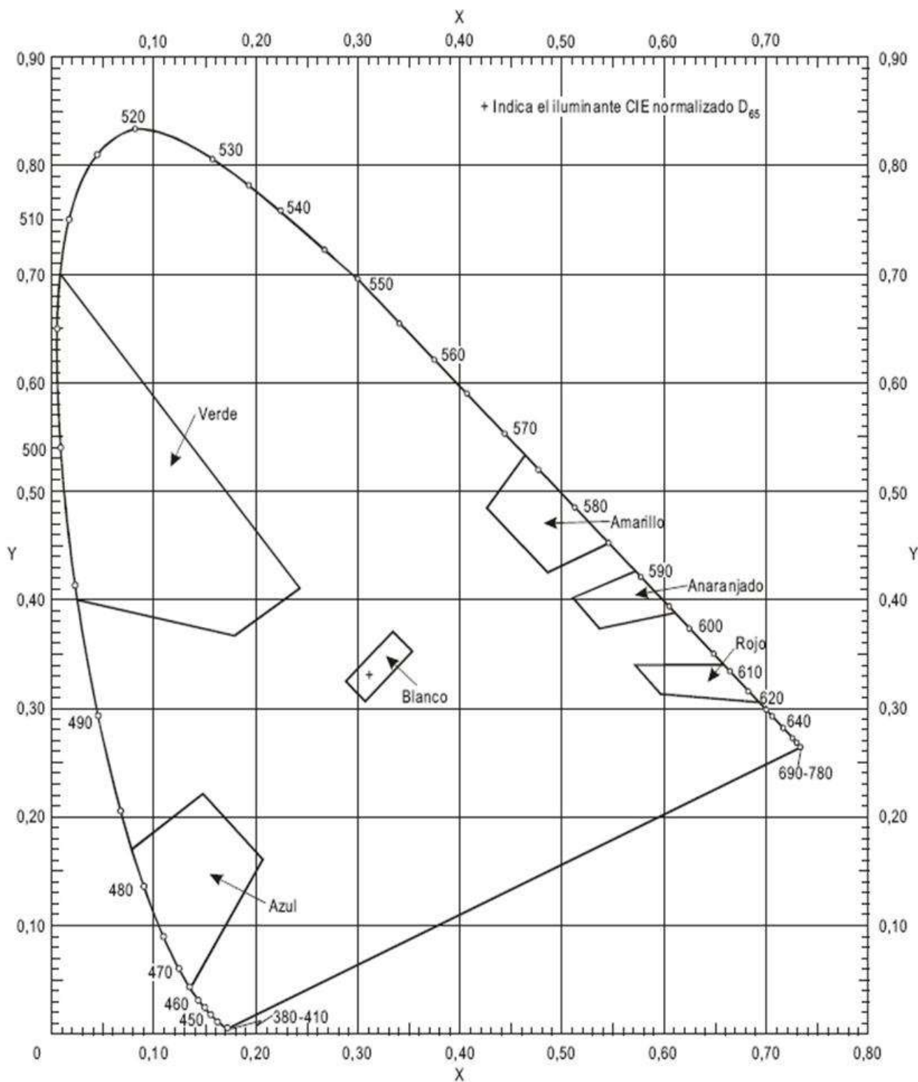
Figura A1-3. Colores de los materiales retrorreflectantes para las señales, letreros y tableros
