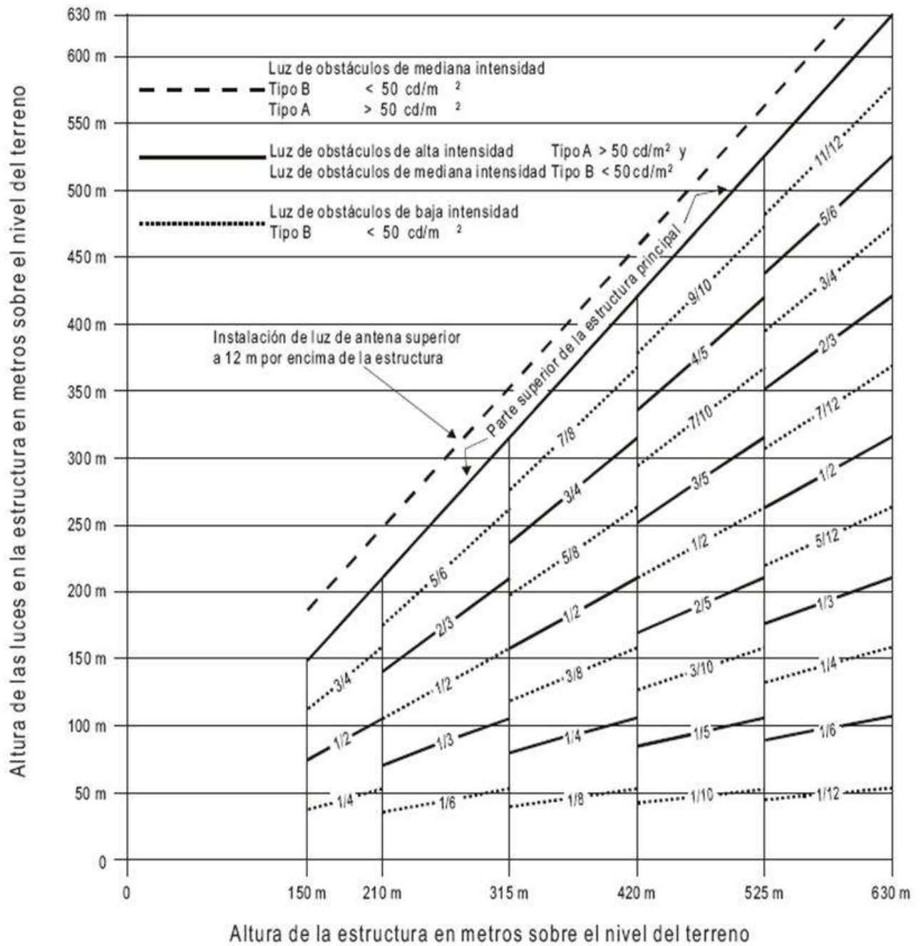
Figura A6-7. Sistema doble de iluminación de obstáculos de mediana/alta intensidad de Tipo A/Tipo B
