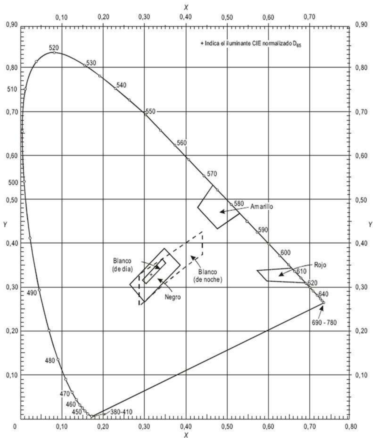
Figura A1-4. Colores de los letreros y paneles transiluminados (iluminación interna)
