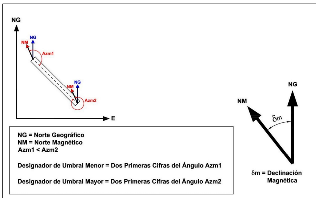
Figura A9-4.- Esquema explicativo para determinación de designador de umbral.
