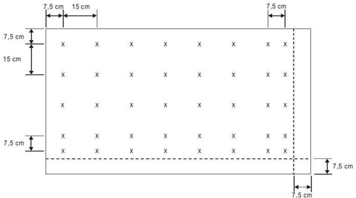
Figura A4-1. Puntos de retícula para calcular el promedio de luminancia de un letrero
