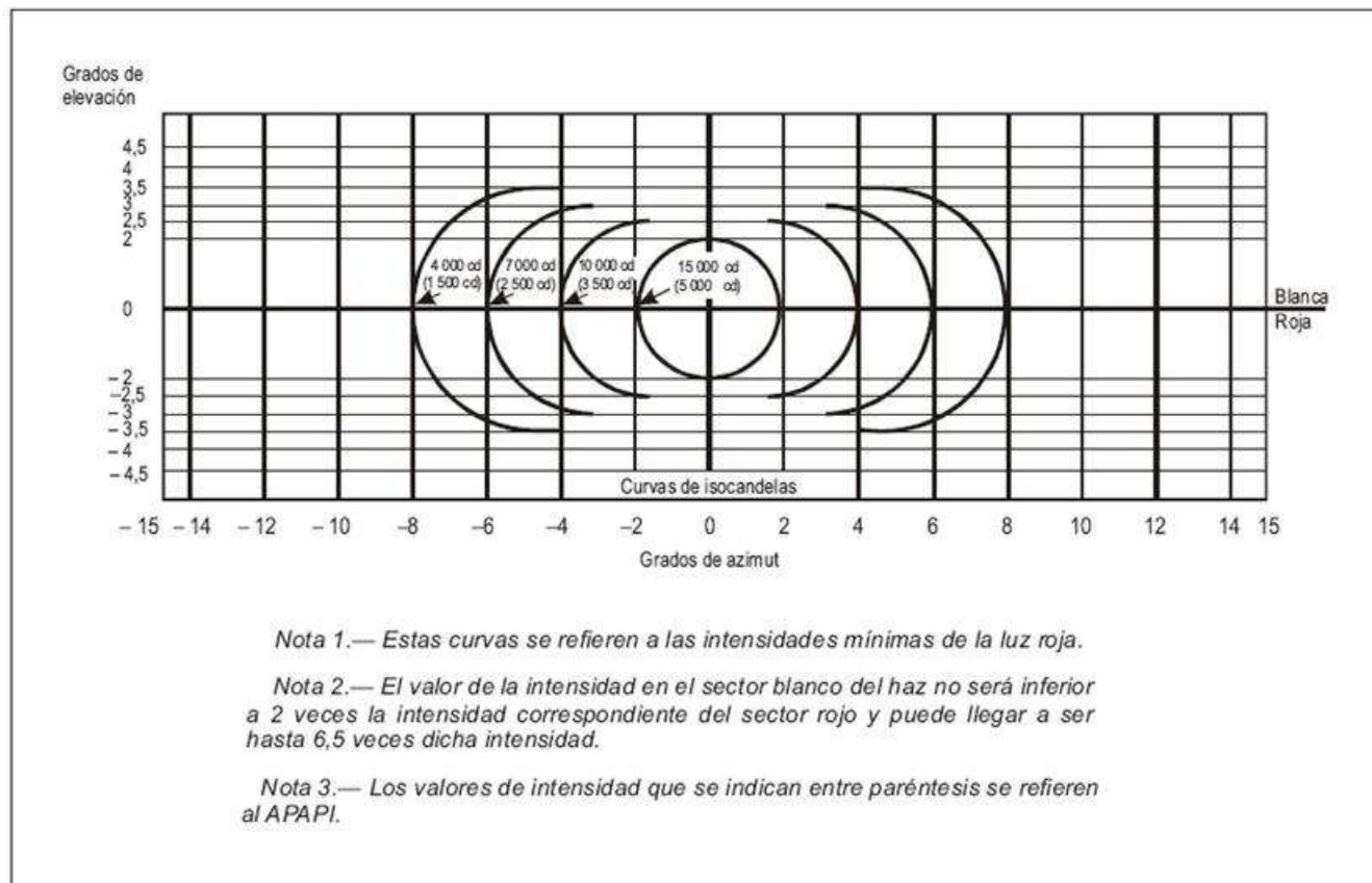
Figura A2-23. Distribución de la intensidad luminosa del PAPI y del APAPI
