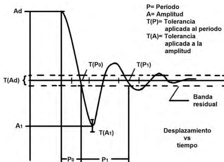
Figura 4.2A Respuesta con amortiguación
