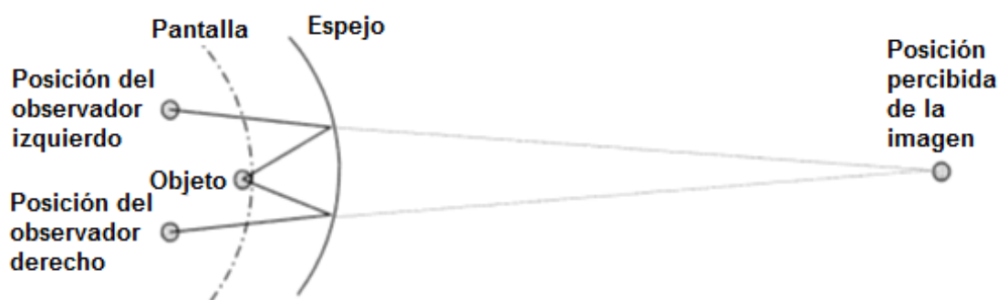
Figura 3.21 Pantalla colimada
