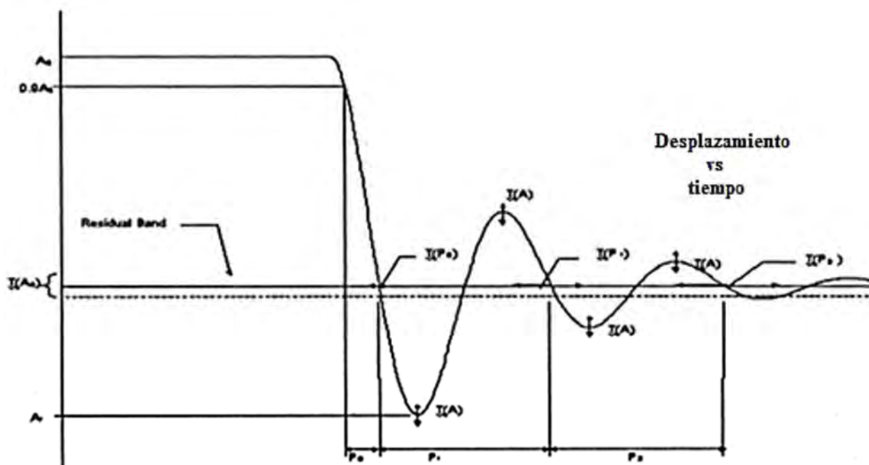
Figura 3.2A Respuesta al movimiento momentáneo de un sistema de baja amortiguación.
