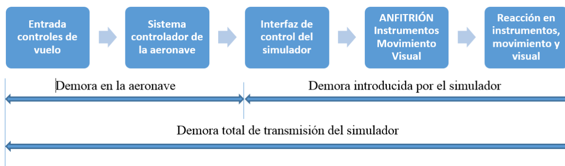
Figura 3.2F Tiempos de transmisión para simulación de aeronaves controladas por computador usando cajas negras reales de helicóptero
