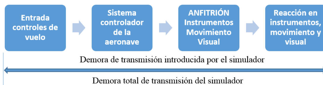
Figura 3.2E Tiempos de transmisión para simulación de aeronaves clásicas no controladas por computador
