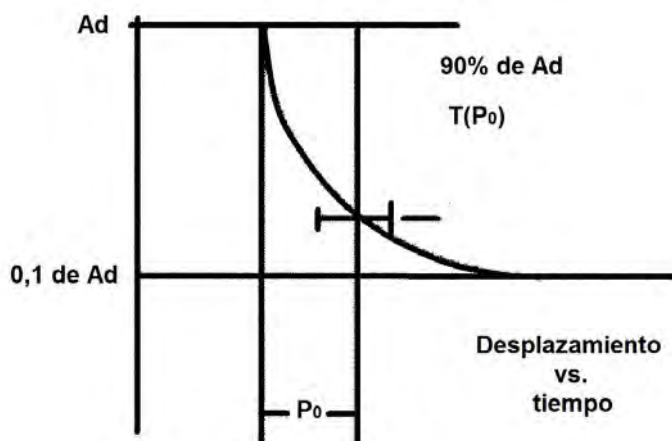
Figura 4.2B Respuesta con amortiguación crítica
