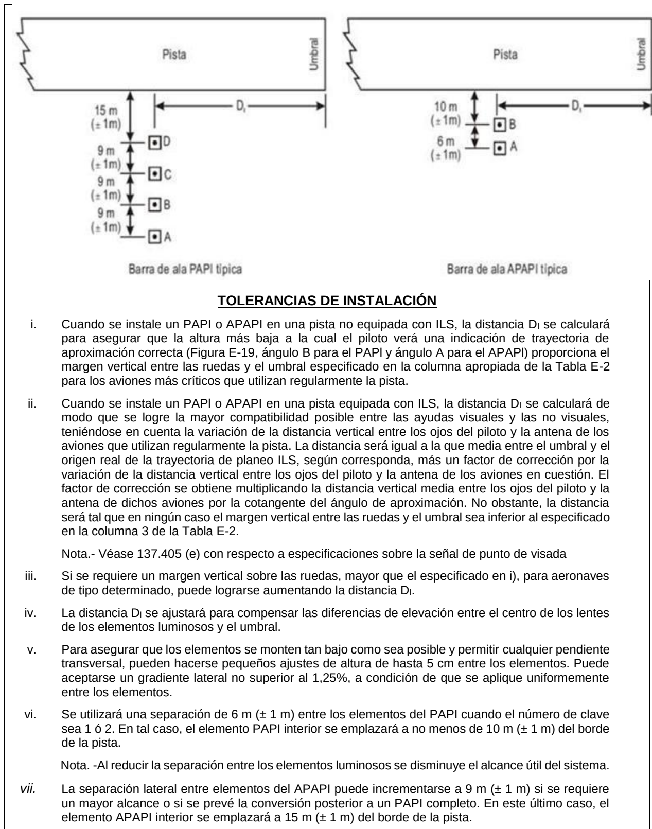
Figura E-20 Emplazamiento del PAPI y del APAPI
