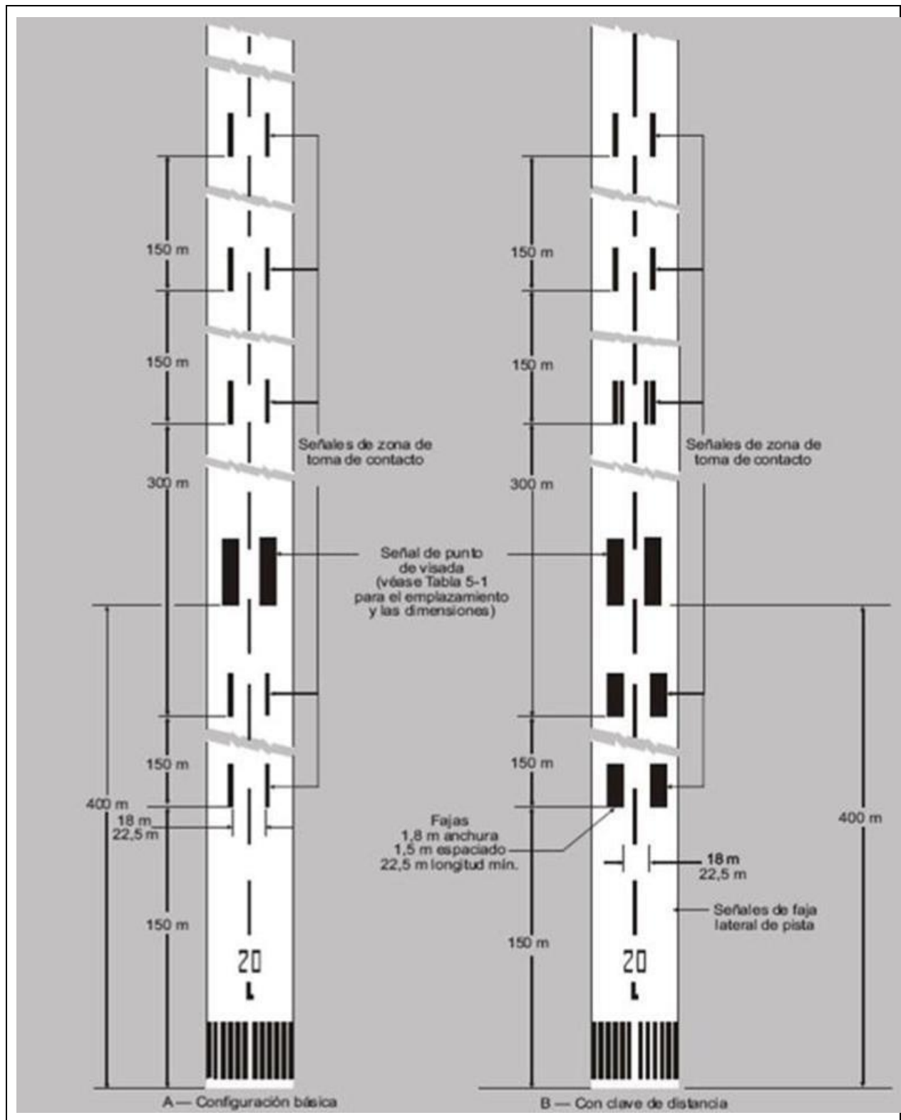
Figura E-5. Señales de punto de visada y de zona de toma de contacto (ilustradas para una pista de 2.400 m de longitud o más)
