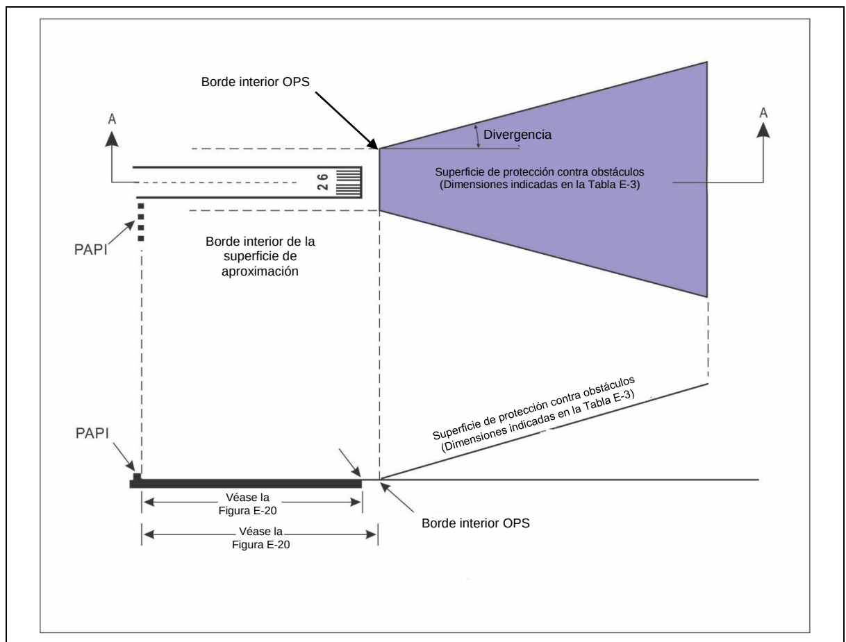
Figura E-22. Superficie de protección contra obstáculos para los sistemas visuales indicadores de pendiente de aproximación
