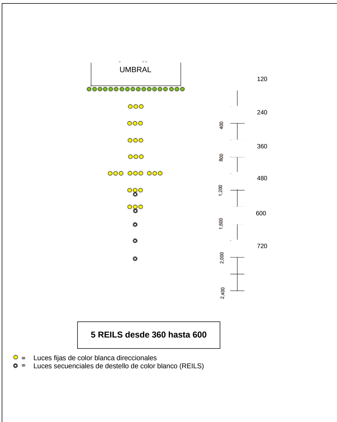
Figura E-17B. Configuración de MALSR reducido (distancias en metros)
