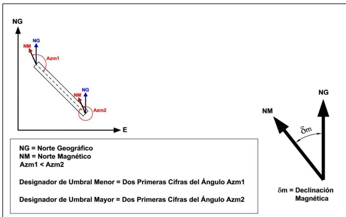
Figura A8-1.- Esquema explicativo para determinación de designador de umbral.
