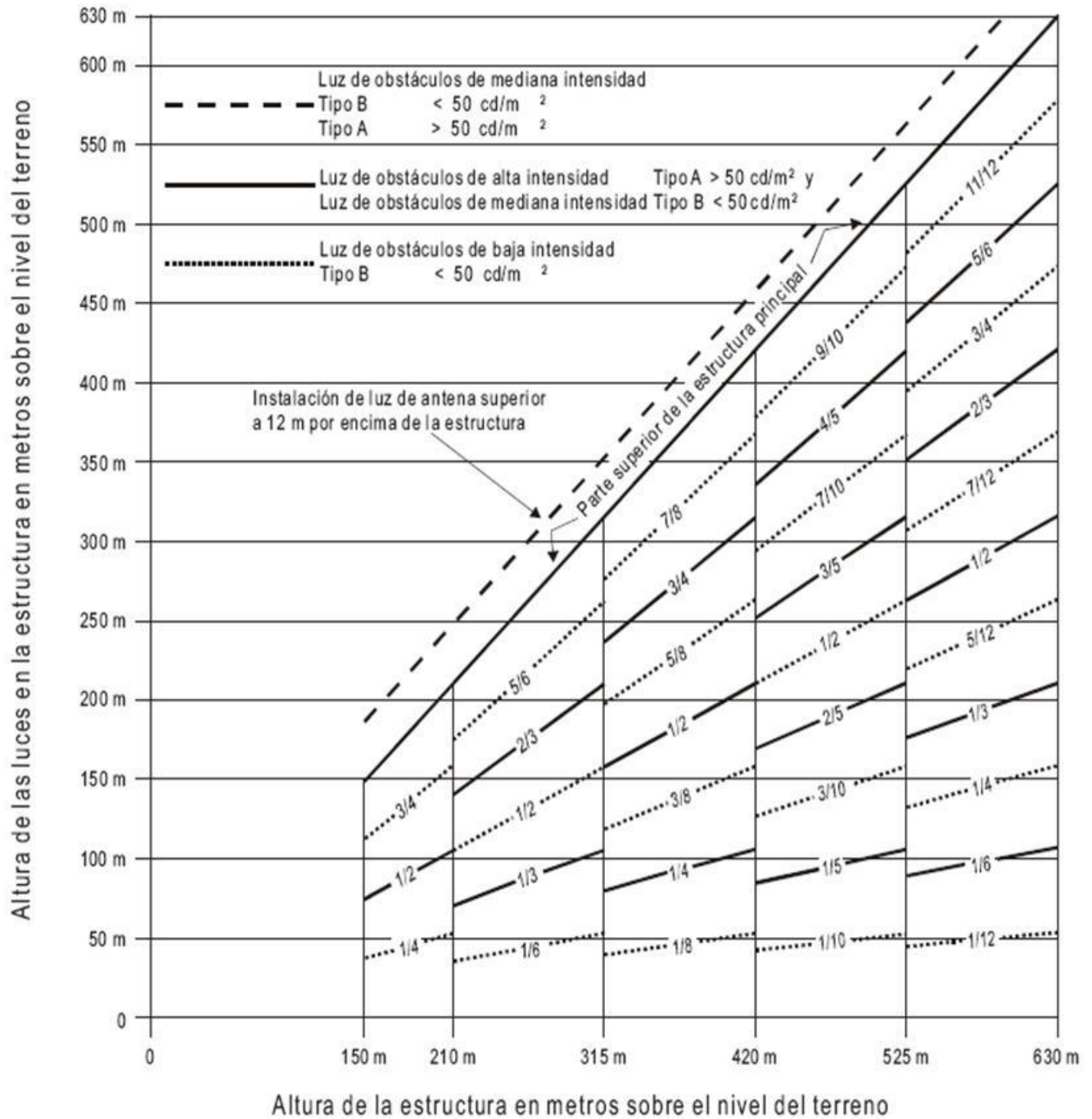
Figura A6-7. Sistema doble de iluminación de obstáculos de mediana/alta intensidad de Tipo A/Tipo B
