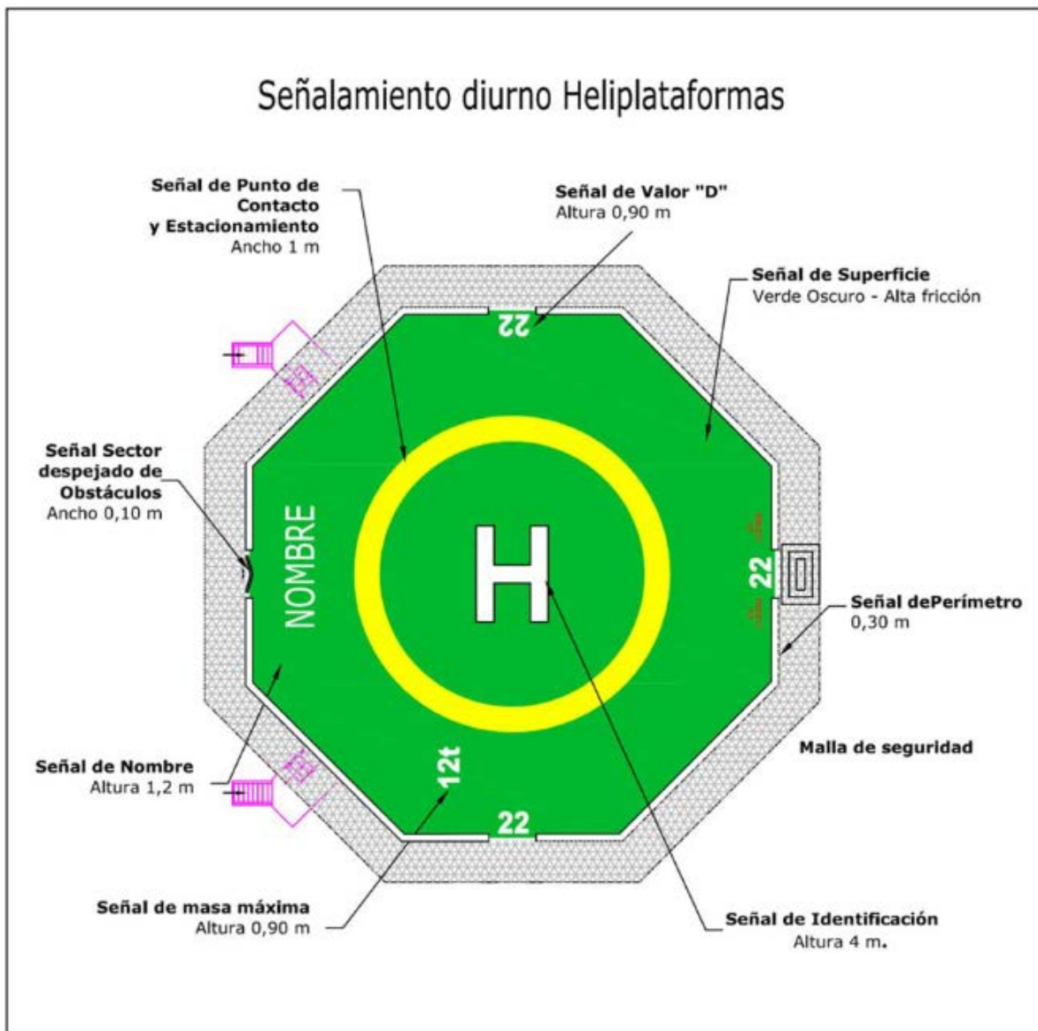
Figura A-5-8. Señalamiento de heliplataporma
