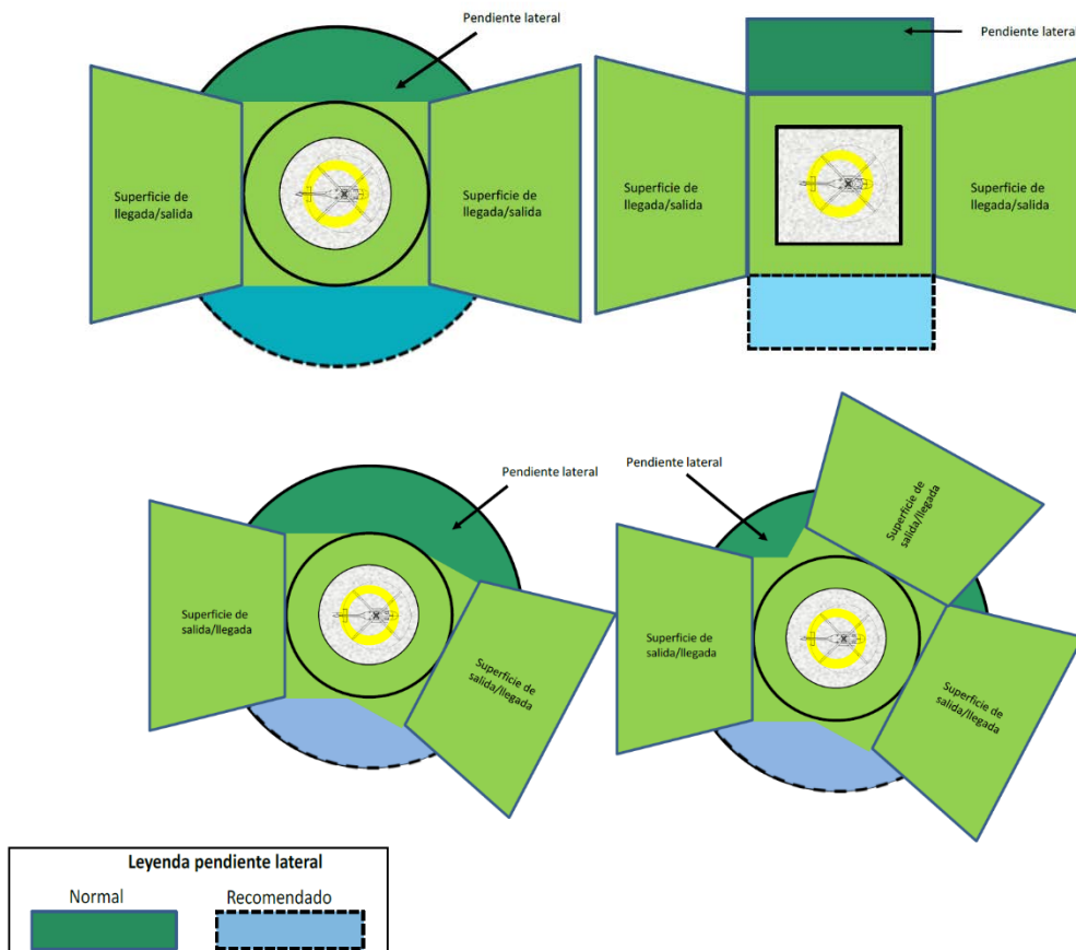
Figura A-3-2. Área de seguridad operacional simple/compleja y pendiente lateral protegida de la FATO
