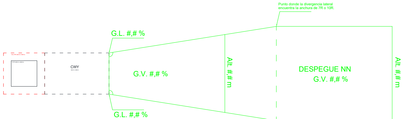
Figura 5-4-13 - Superficie de Ascenso en el Despegue
